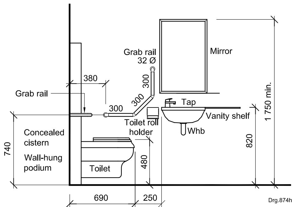
Elevation A-A
