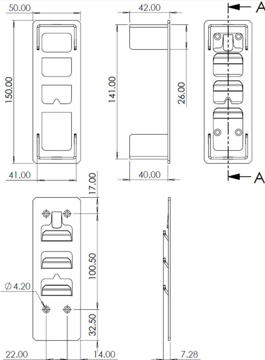
SECTION A-A
